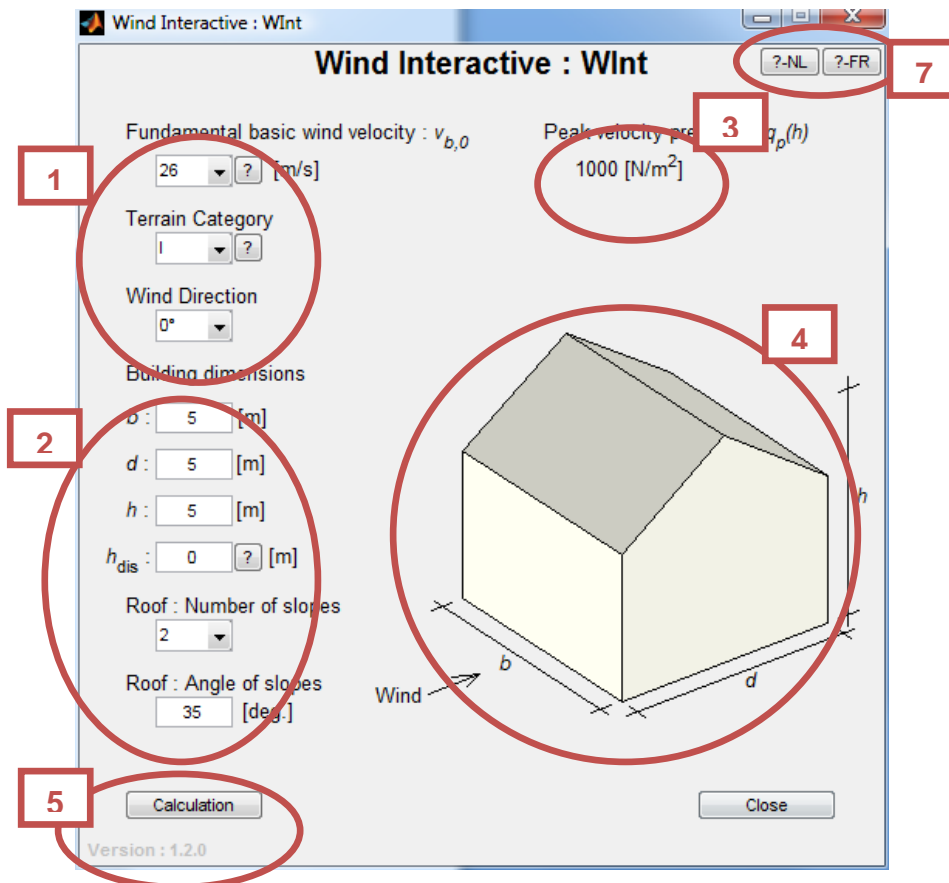
Figure 1 : Fenêtre principale
